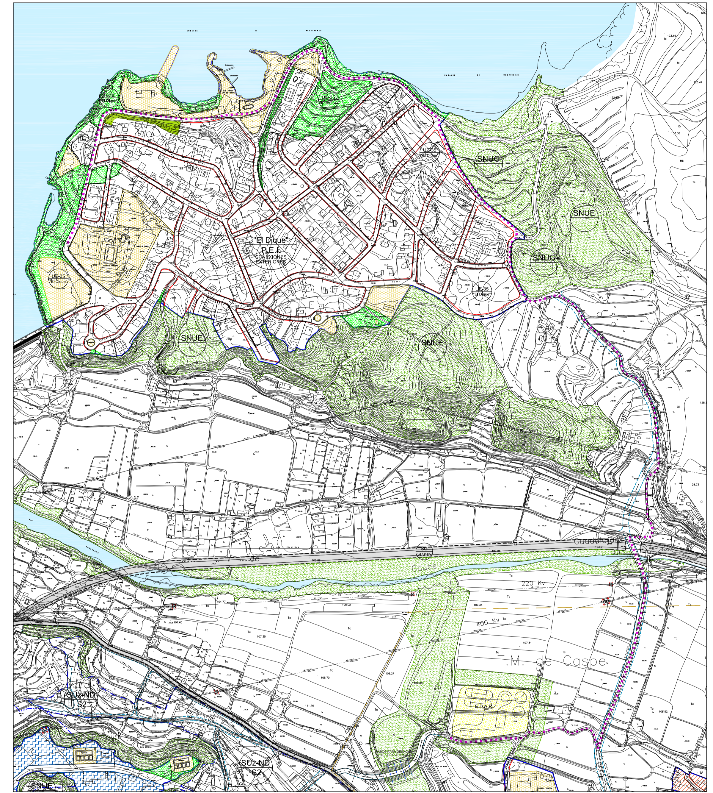
COLECTOR PROYECTADO Escala: 1/4.000
